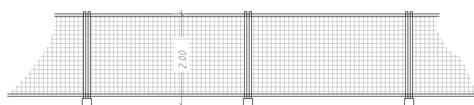
Particolare recinzione scala 1:100
